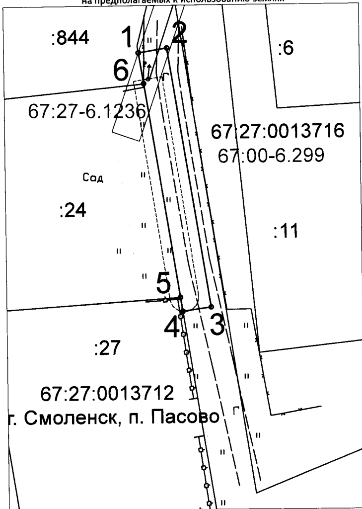
ЧЕРТЁЖ РАЗМЕЩЕНИЯ ОБЪЕКТА на предполагаемых к использованию землях
